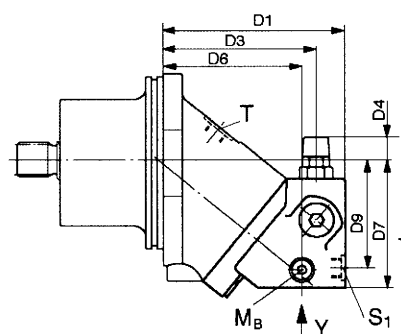
Detail Y
