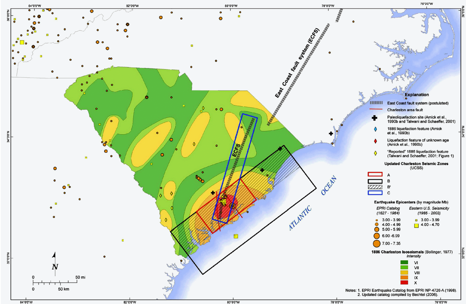
Figure 2.5-56—{UCSS Map}
