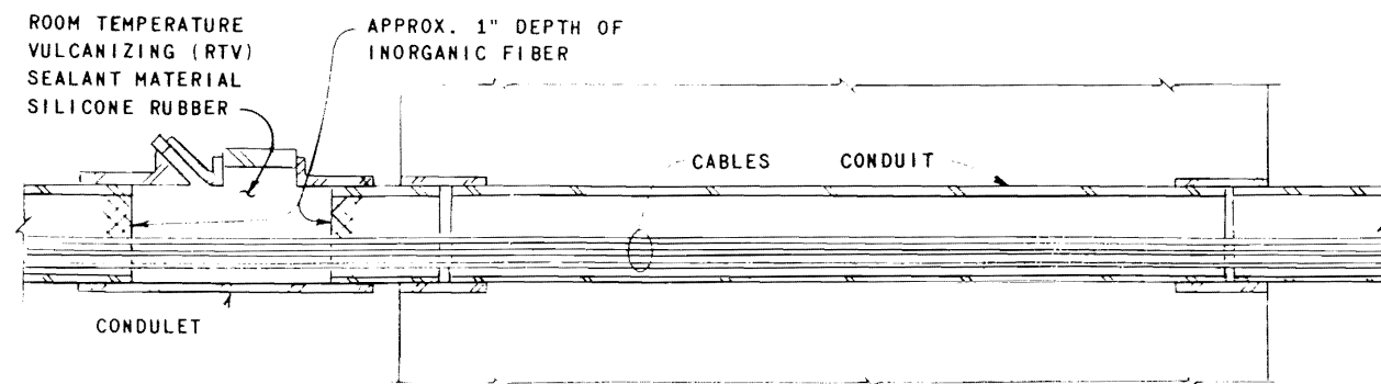
CONDUIT PENETRATION
