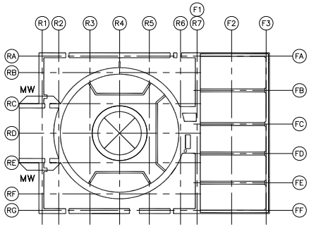
FLOOR EL 17500
