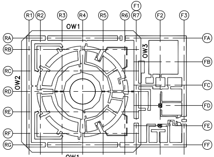
FLOOR EL -11500
