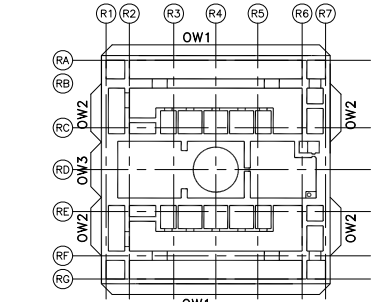
FLOOR EL 27000
