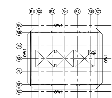
FLOOR EL 34000
