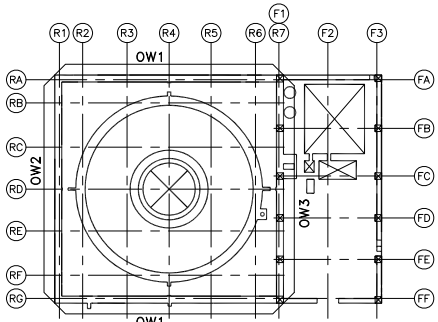
FLOOR EL 4650
